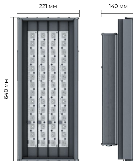
Ямал 160-240 Вт
