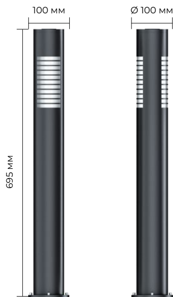
Столбик П (АЗДФ закладная)
