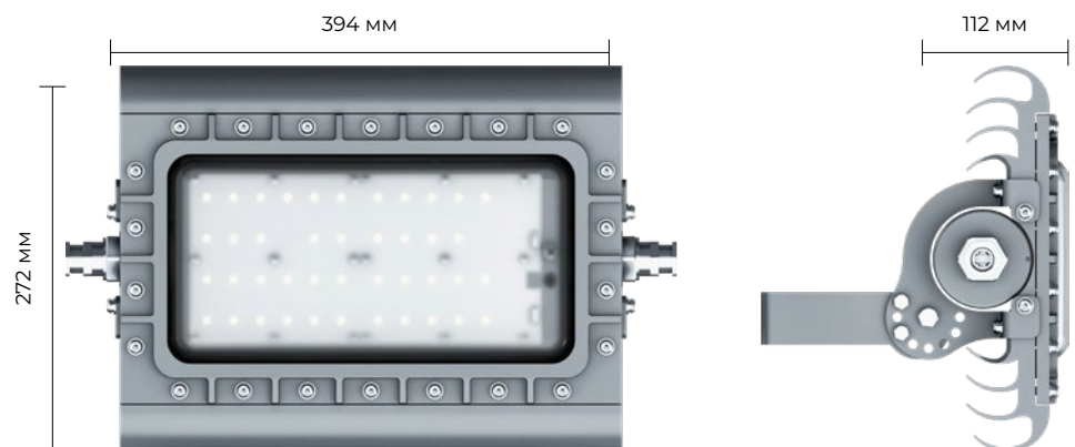
PROEX 100–120 Вт
