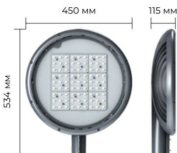
На кронштейн
